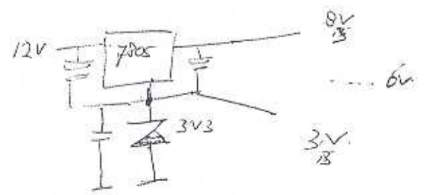
SPANNING T.B.V. DITTE DECODEE (UITGANG VERLEEDT TUSSEN 3V3 EN 8V3 ↓ ↓ LAGE HOOG
